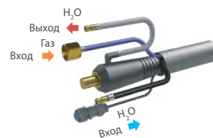
ОКС, M10x1 (вход газ), 6/р (выход H 2 O, вход H 2 O), 7 pin
