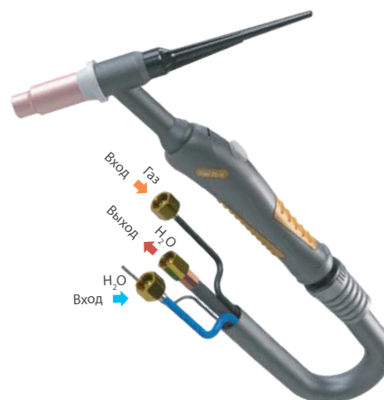
M12x1 (выход H 2 O), 1/4G (вход газ), 3/8G (вход H 2 O)
